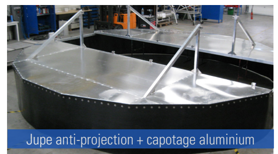
Capotage d'insonorisation
