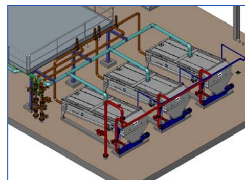
Conjunto de 3 Mesas Espesadoras OMEGA 15 LD
